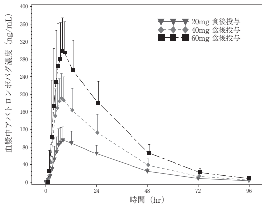
図1 食後単回経口投与時の血漿中アパロンボパグ濃度推移（健康成人）（算術平均＋標準偏差）
