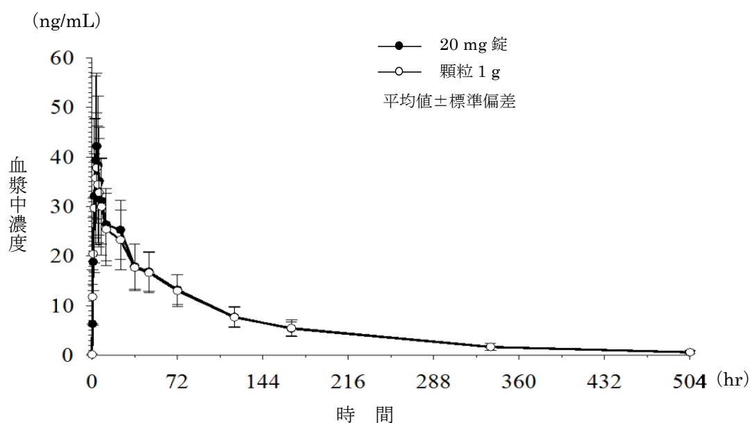
図Ⅶ-2 20 mg 錠又は顆粒 1 g (パロキサビル マルボキシルとして 20 mg) の単回経口投与時のパロキサビル マルボキシル活性体の平均血漿中薬物濃度推移 (算術平均)
