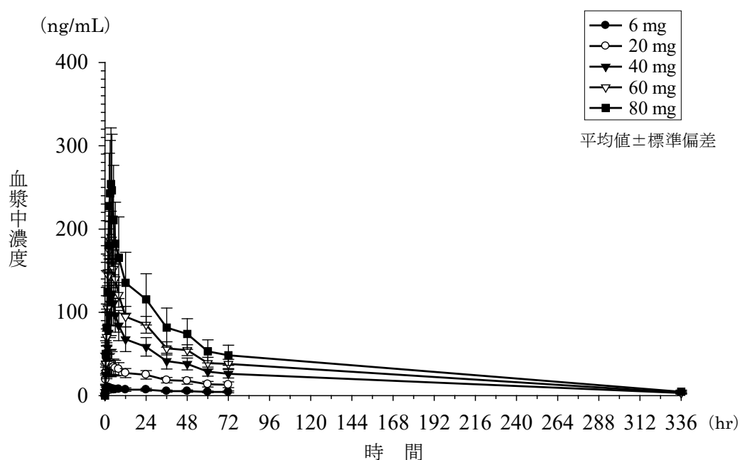
図VII-1 パロキサビル マルボキシル空腹時単回経口投与時の平均血漿中パロキサビル マルボキシル活性体濃度推移
