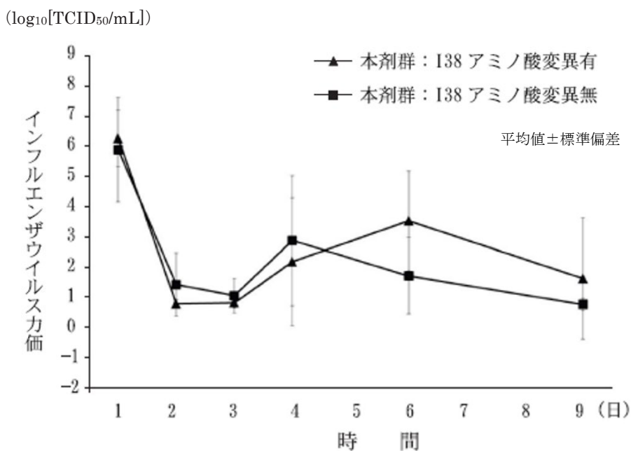
図VI-19 小児患者対象第Ⅲ相臨床試験（顆粒剤）（T0833）におけるポリメラーゼ酸性蛋白質領域の I38 アミノ酸変異の有無別のウイルス力価の推移
